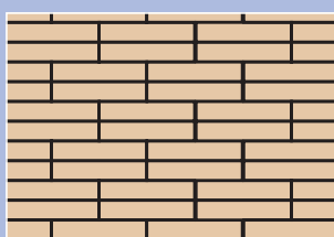
Englischer Verband (doppelt)
